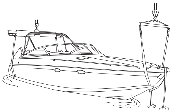
1. Spreader Bar
